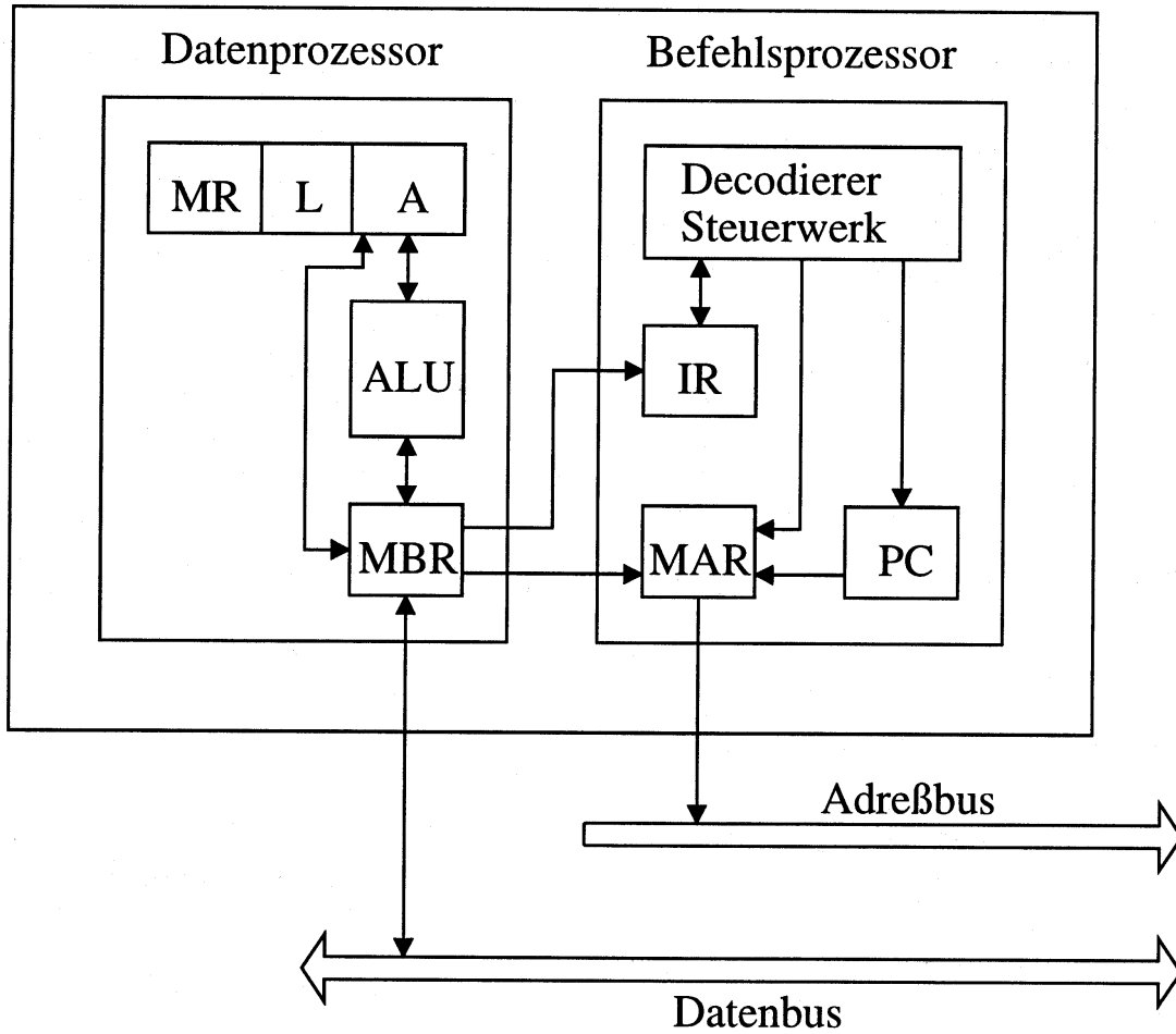
Abbildung 1: Struktur einer CPU
