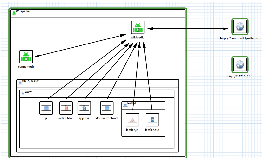
Abb. 4: Grafische Darstellung der Zwischendarstellung.
