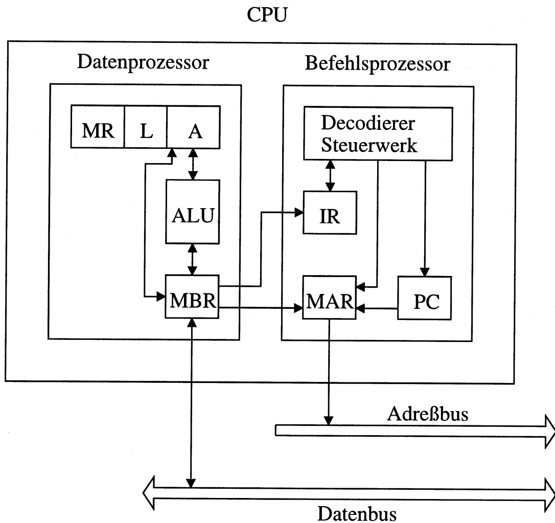
Abbildung 1: Struktur einer CPU
